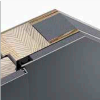
Composition bois mousse thermique / aluminium pour une isolation thermique maximale
